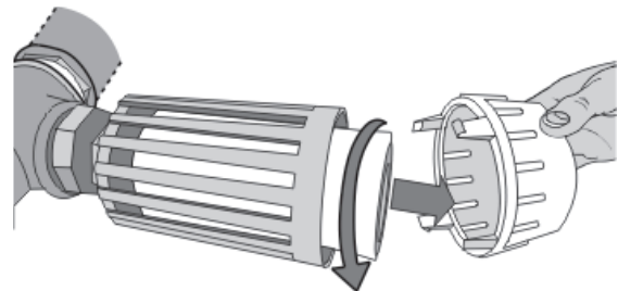
Schalldämpferelement erneuern
